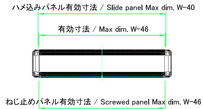
A-A (1:8)
